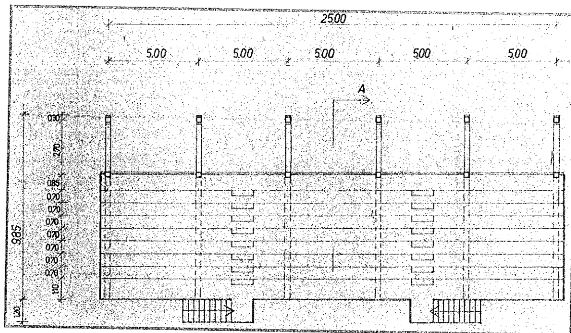
Pianta della tribuna
