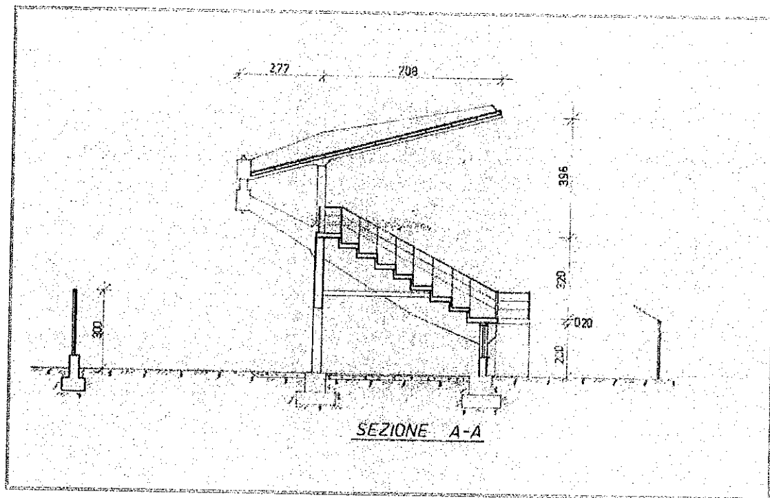
Sezione della tribuna
