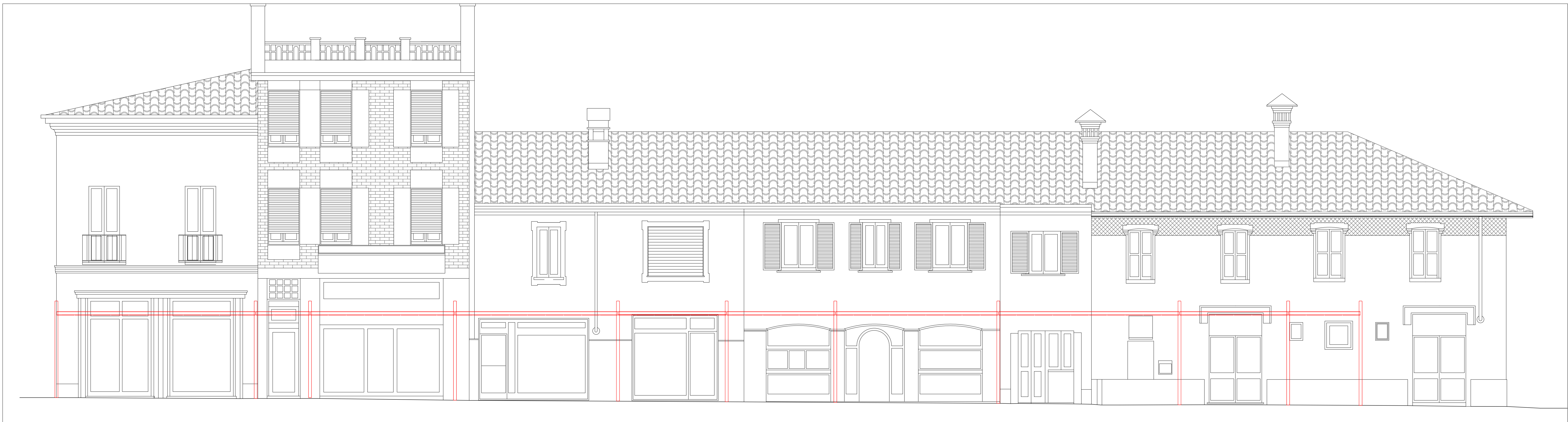
PROSPETTO OVEST | TRATTO A (comparativa) - 1:50
