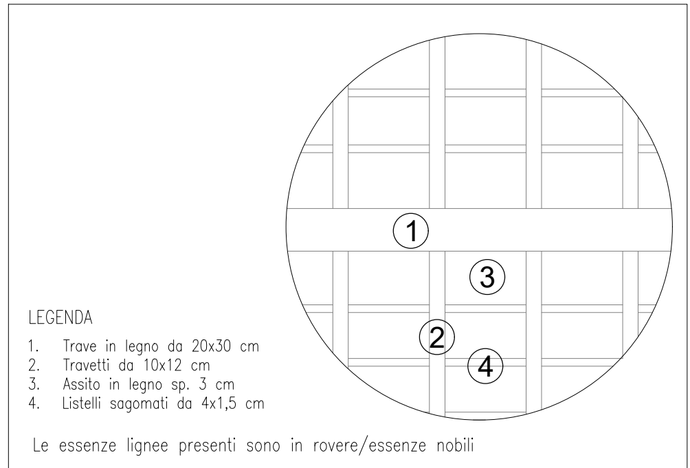
DETTAGLIO TIPO PIANTA SOLAI IN LEGNO
