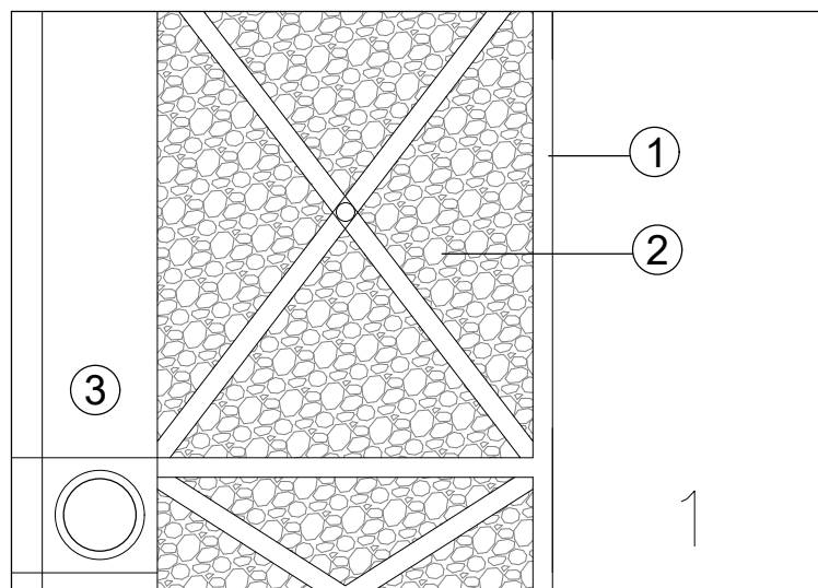
1- Particolare pavimentazione
