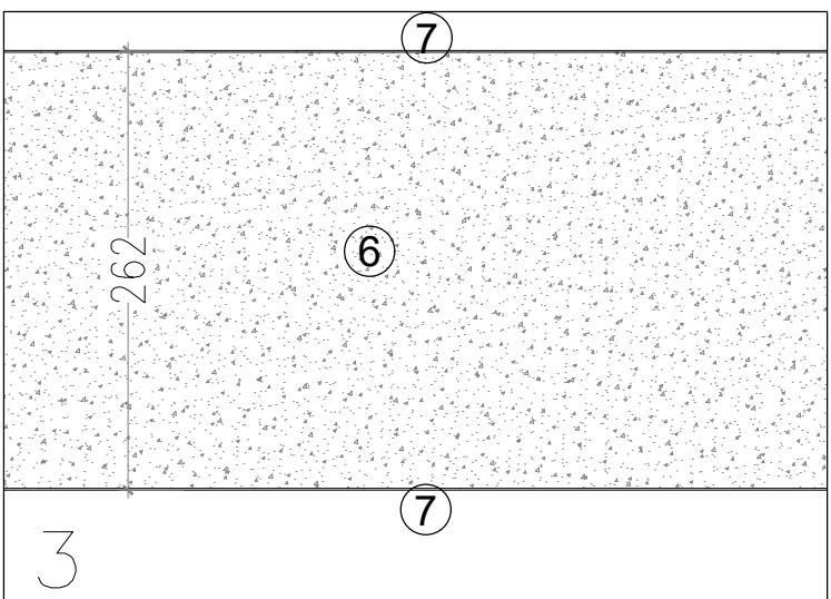
3- Particolare nuova pavimentazione
