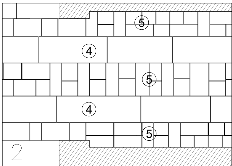
2- Particolare pavimentazione
