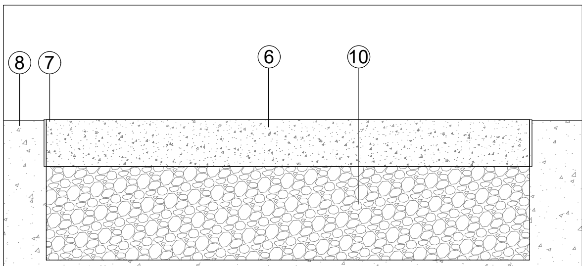
4- Particolare sezione nuova pavimentazione
