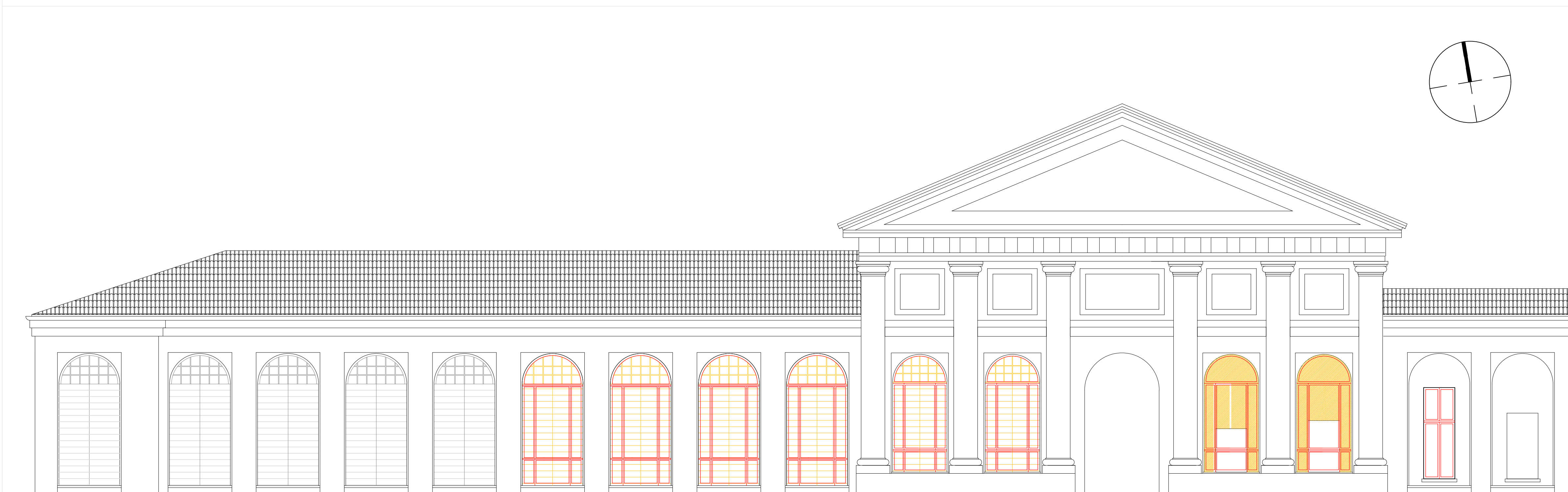
Prospetto serre
