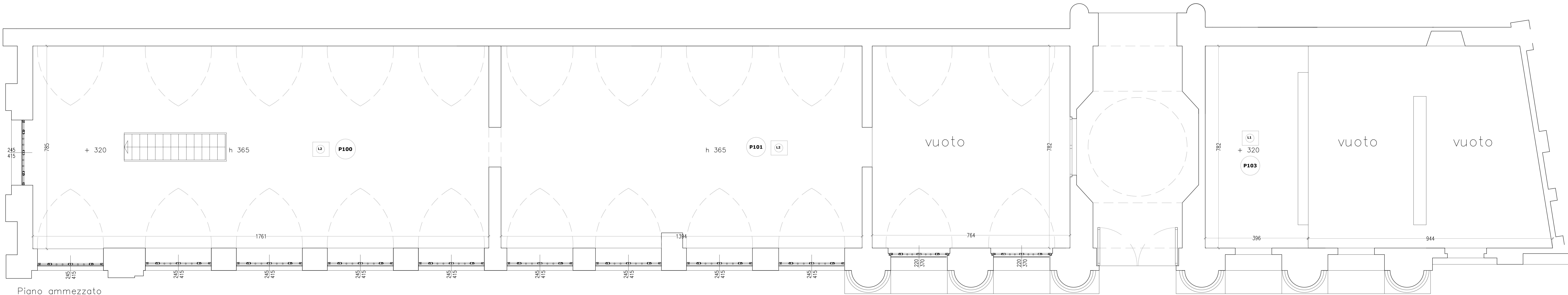
Piano ammezzato
