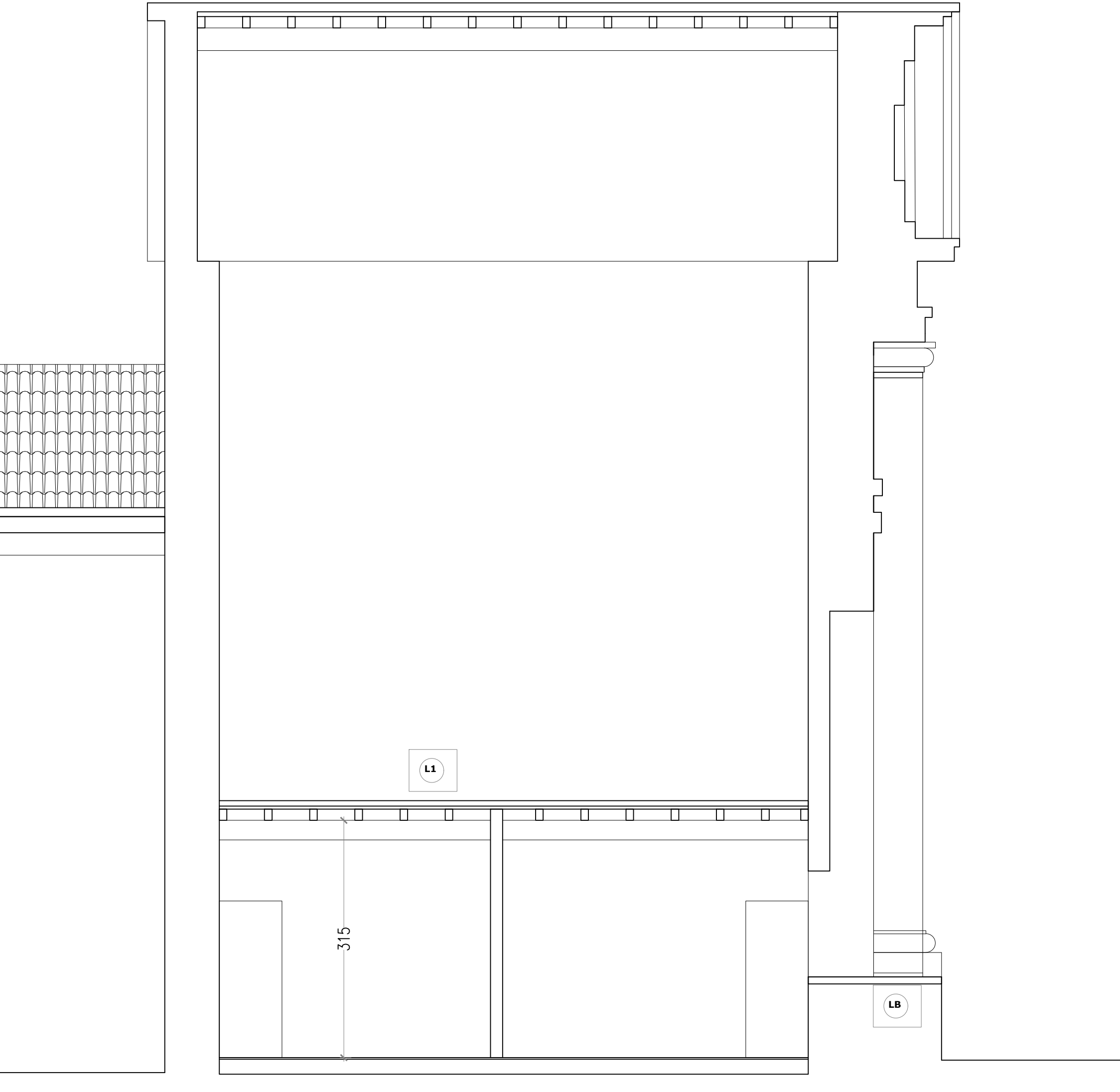
Sezione B-B trasversale corpo ingresso oggetto di recupero
