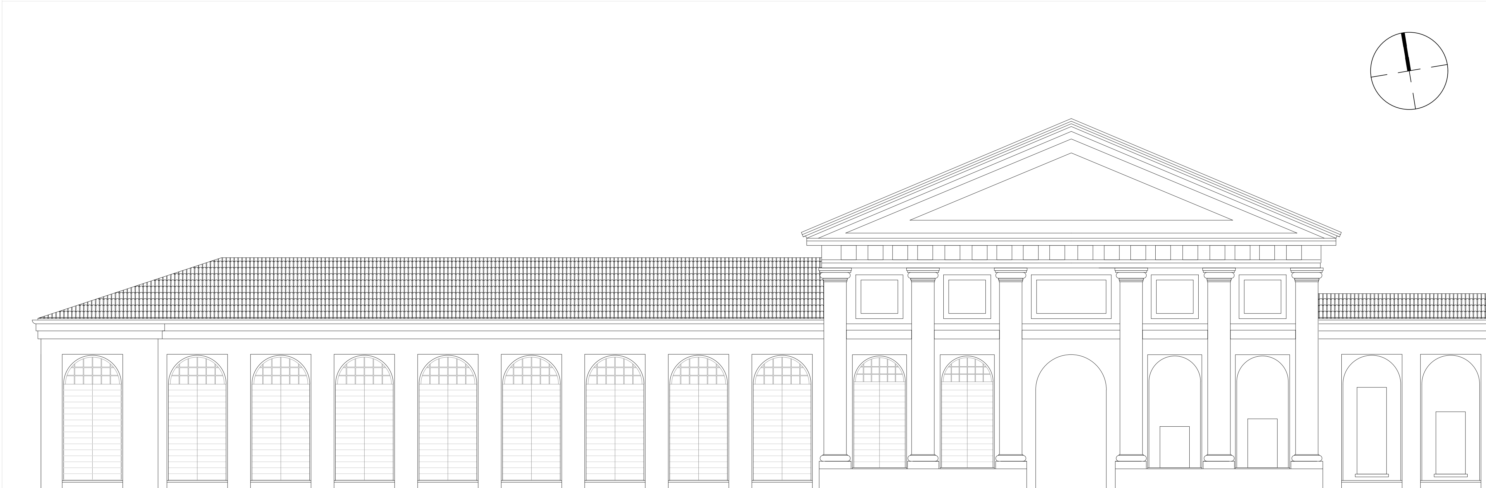
Prospetto serre
