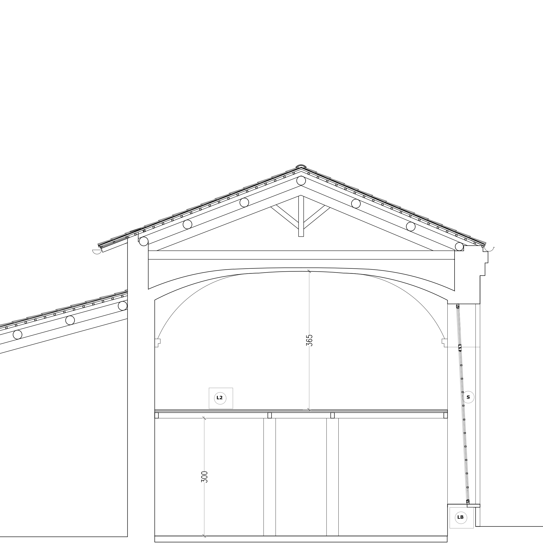
Sezione A-A trasversale corpo serre con recupero al rustico
